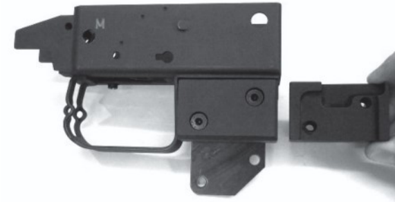
Figura 30: adattatore per l’impugnatura per F ass 57
