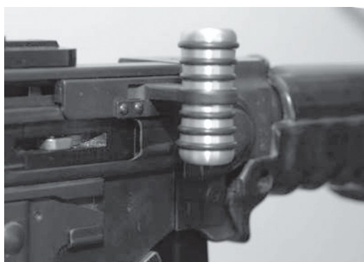
Bild 34: Ladegriff anatomisch zu Stgw 57
