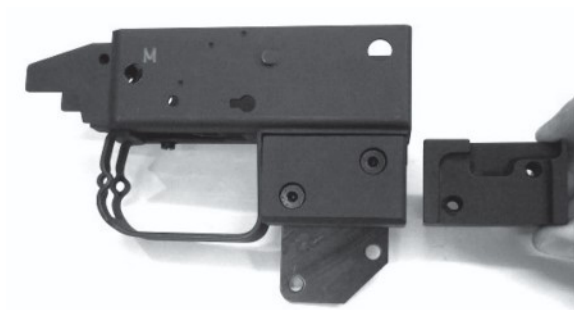
Bild 30: Griffadapter zu Stgw 57
