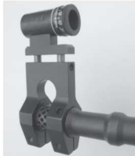
Bild 26: Korntreger als Visierverlängerung (Montage auf Mündungsbremse), diverse Fabrikate
